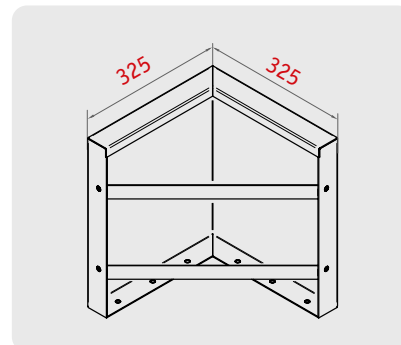
Außenecke
